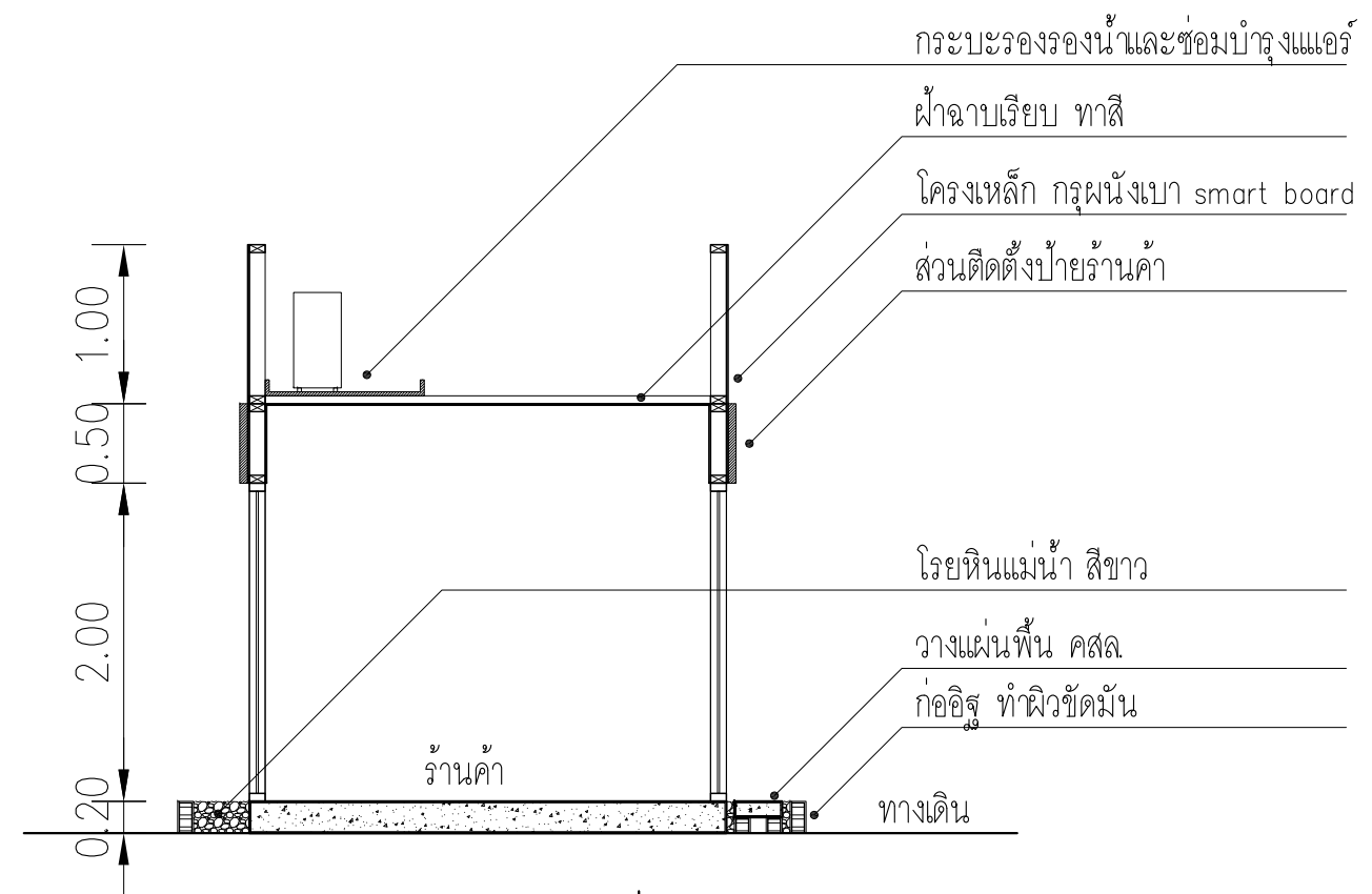
รูปตัด A-A 1:50
