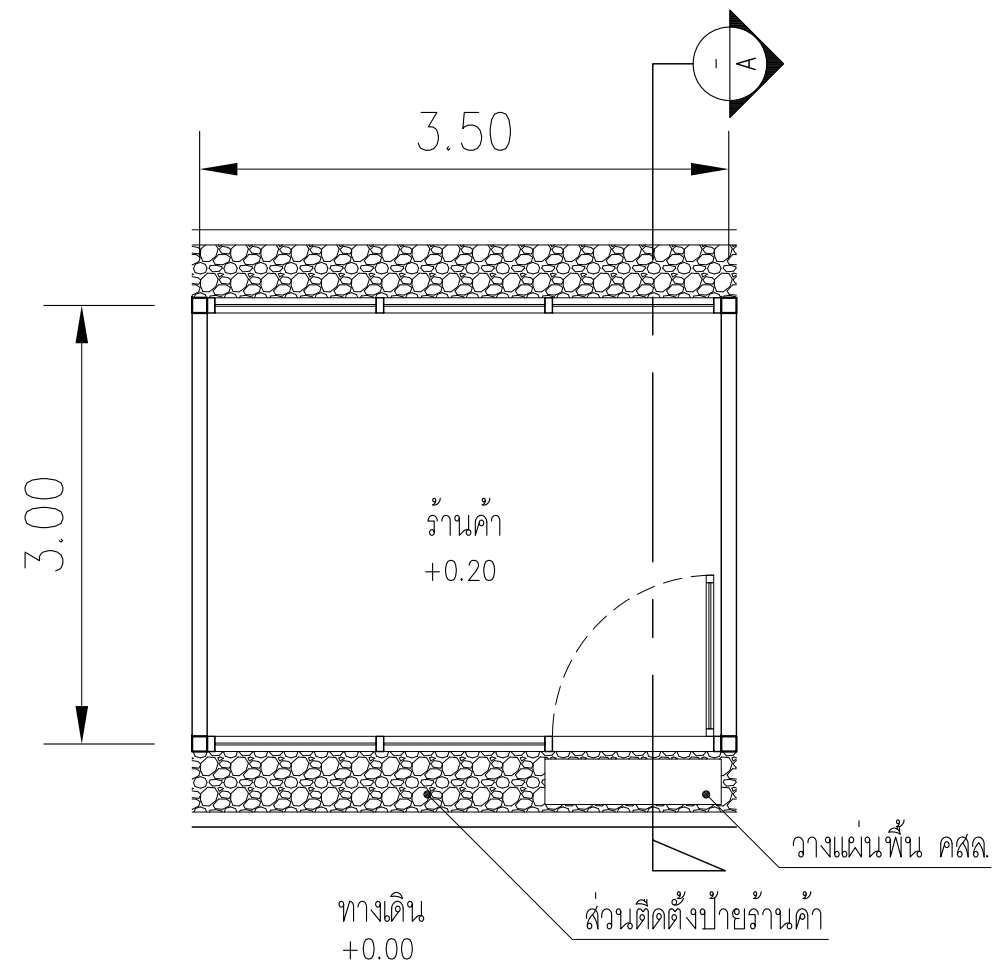
แปลนร้านค้า 1:50
