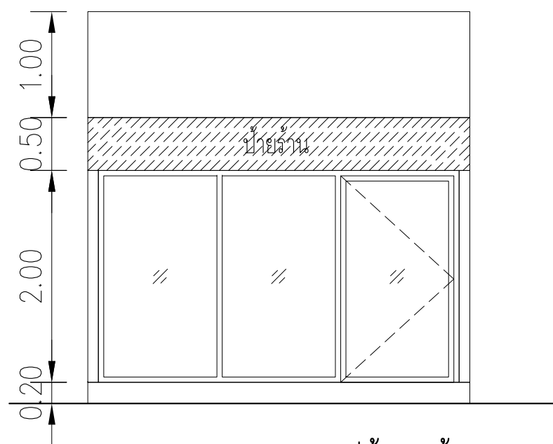
รูปด้านหน้า 1:50
